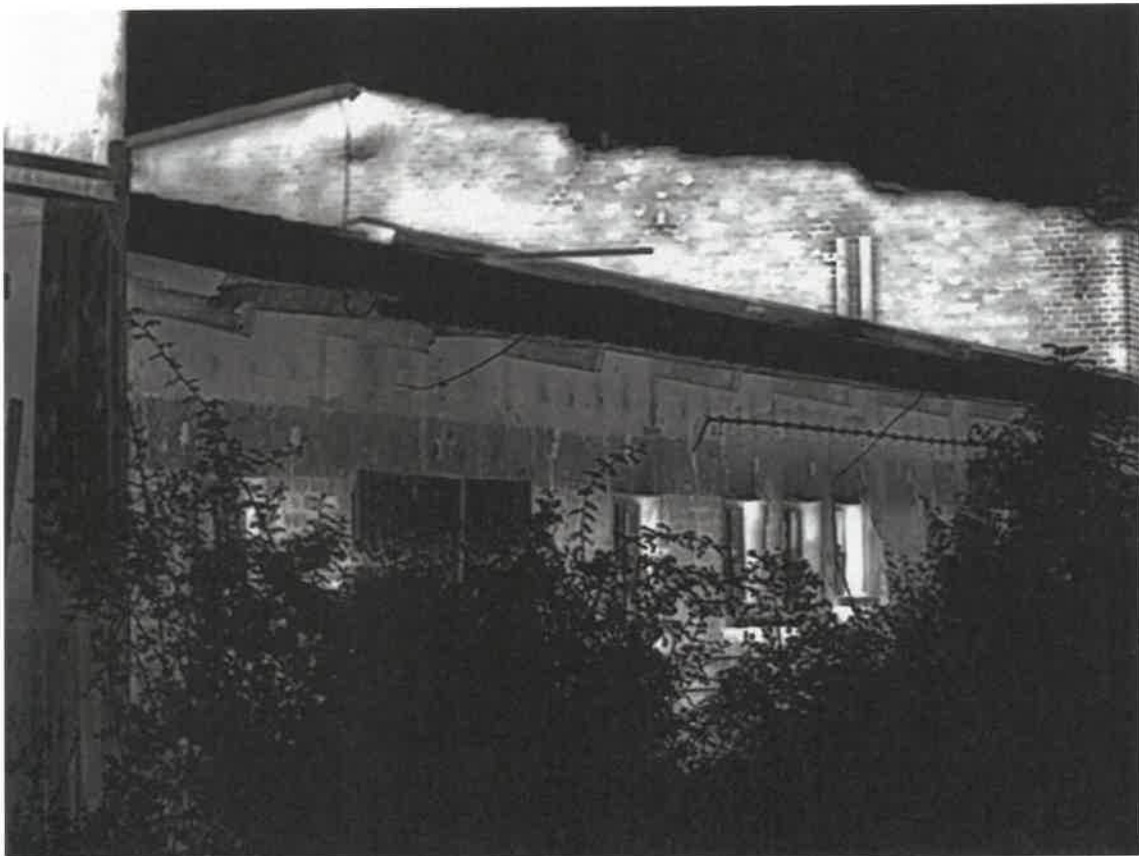
Abbildung 49: Südwestseite von Gebäude 1 im Wärmebild.
