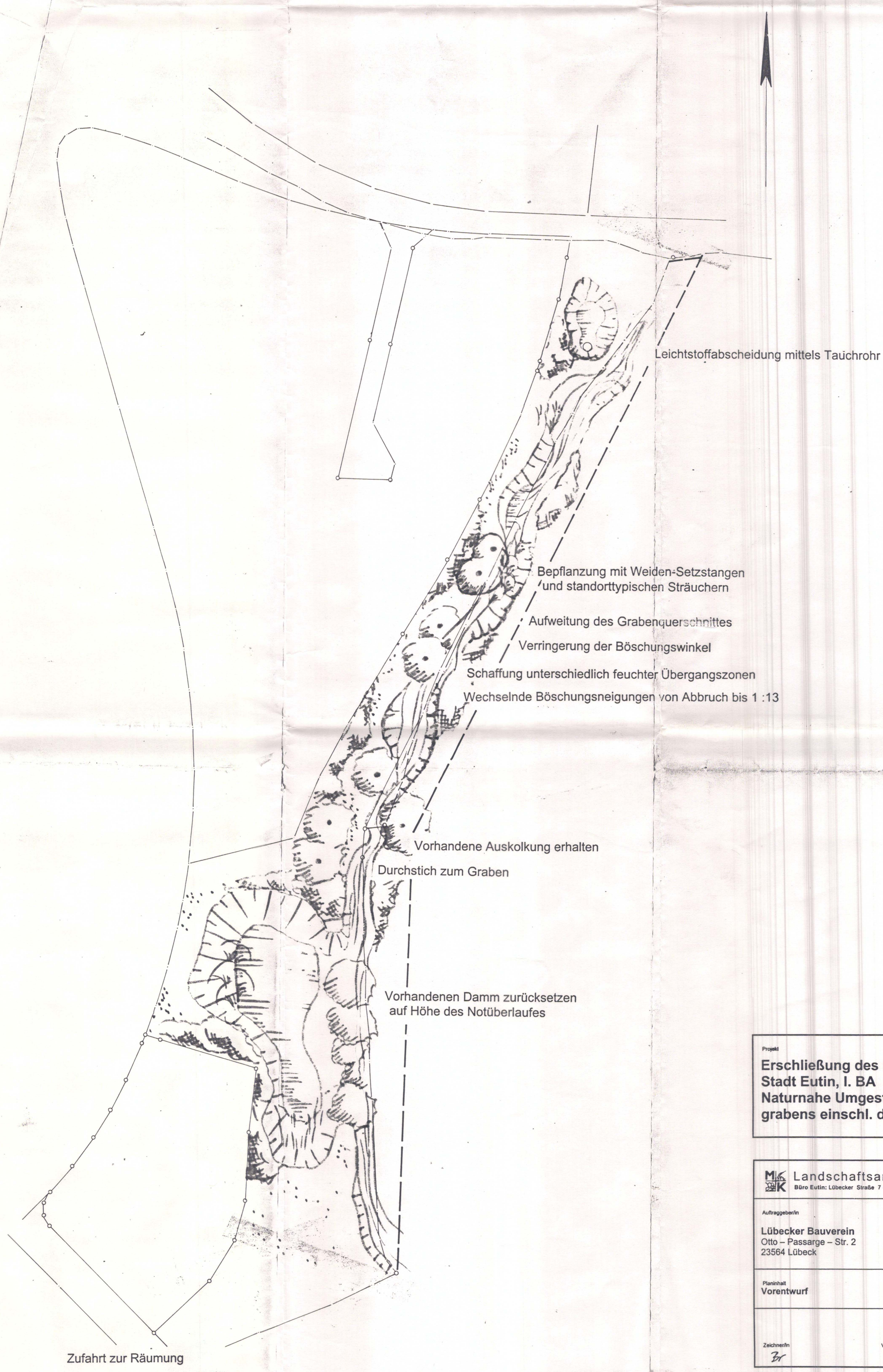
Detailplanung zur „Naturnahen Umgestaltung des Ehmbruchgrabens einschließlich Regenrückhaltebecken“ (MÜLLER & KAHNS Aug. 2000)
